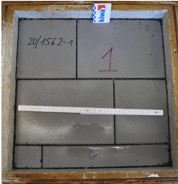
Abbildung 1: Pflastersteine mit Fugenmaterial in der Form verlegt (nach der Prüfung)
