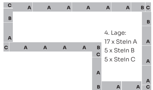
Höhe: 0,60 m
