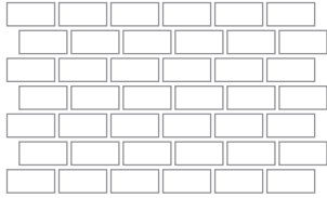
Stein 24/12/8 cm: Versatz um 6 cm
